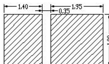
建议焊盘
